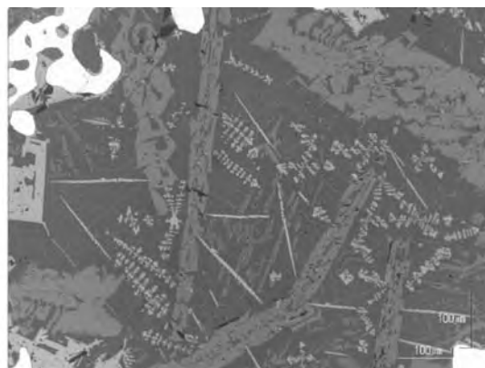
(b) 鉄塊 1 スラグ部分
