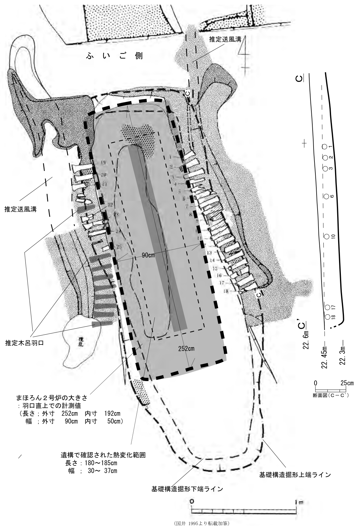
図14 まほろん2号炉の炉壁厚と15号製鉄炉
