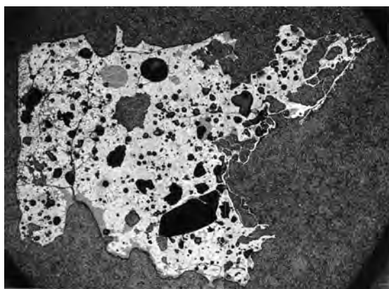
写真 26 マクロ写真 (NO. 1) × 5
