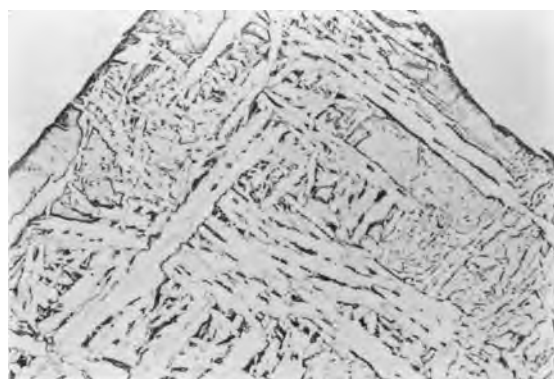
写真 60 鉄組織写真（資料 NO. 7-1）× 400
