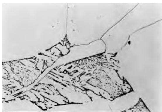
写真 62 鉄組織写真（資料 NO. 7-2）× 400
