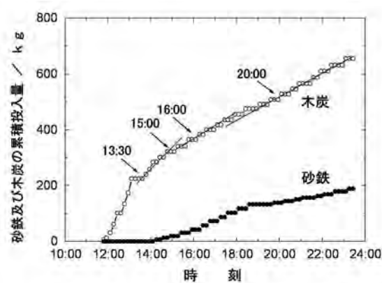
図 4 砂鉄と木炭の累積投入量
