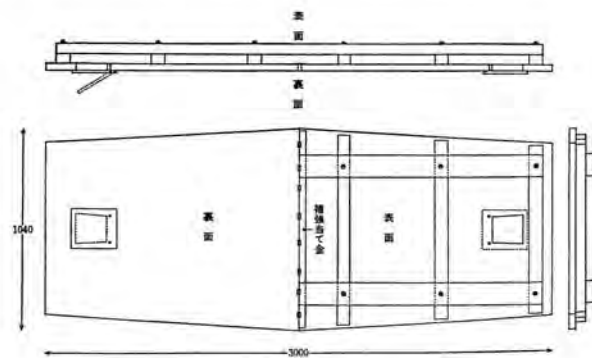
踏み鞆の踏み板（京都市，高橋鋳工場蔵）
