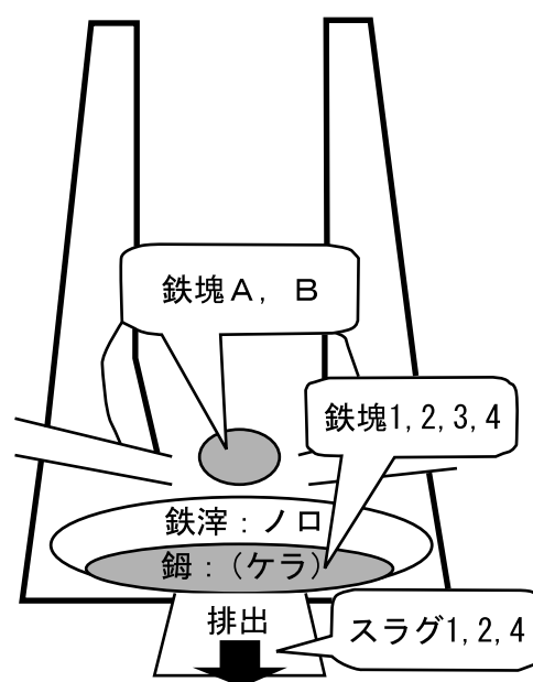
図 1 分析試料の採取場所
