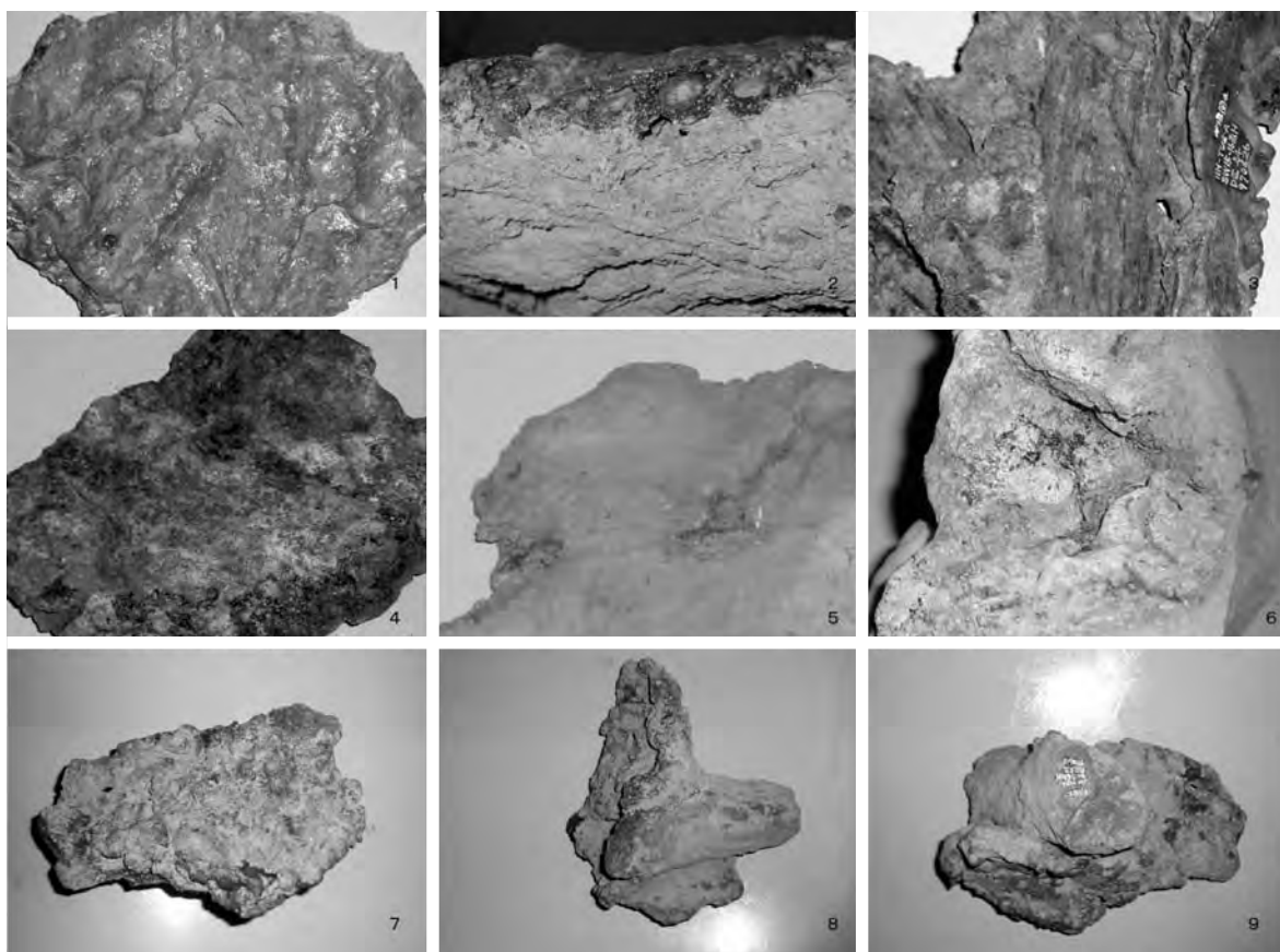
鳥打沢 A 15・16 号 1 炉壁内面 2 炉壁断面 3 発泡滓木炭痕 大迫 5 号 4 炉壁内面 5 炉壁裏側 6 送風孔側面 鳥打沢 A 15・16 号第 12 図 13 7 炉壁内面 8 側面 9 裏側（1～3、7～9 原町Ⅸ、4～6 原町Ⅷ）
