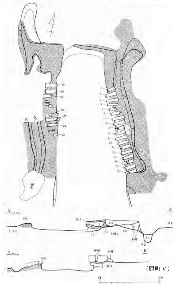
2 大迫A15号羽口設置状況
