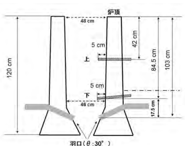
図 1 炉の断面図と熱電対の設置位置
