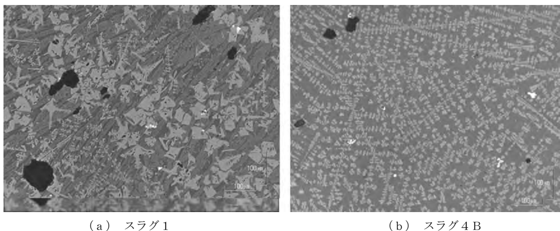
図8 製鍊滓試料の光学顕微鏡観察像
