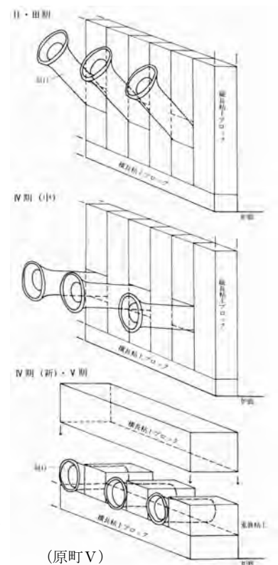
図6 小暮伸之による羽口装着案
