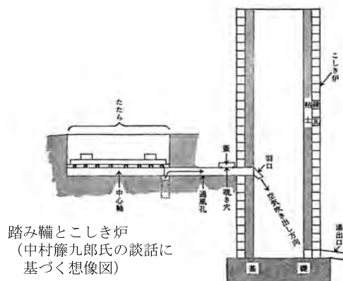
図6 参考にした踏み鞆
