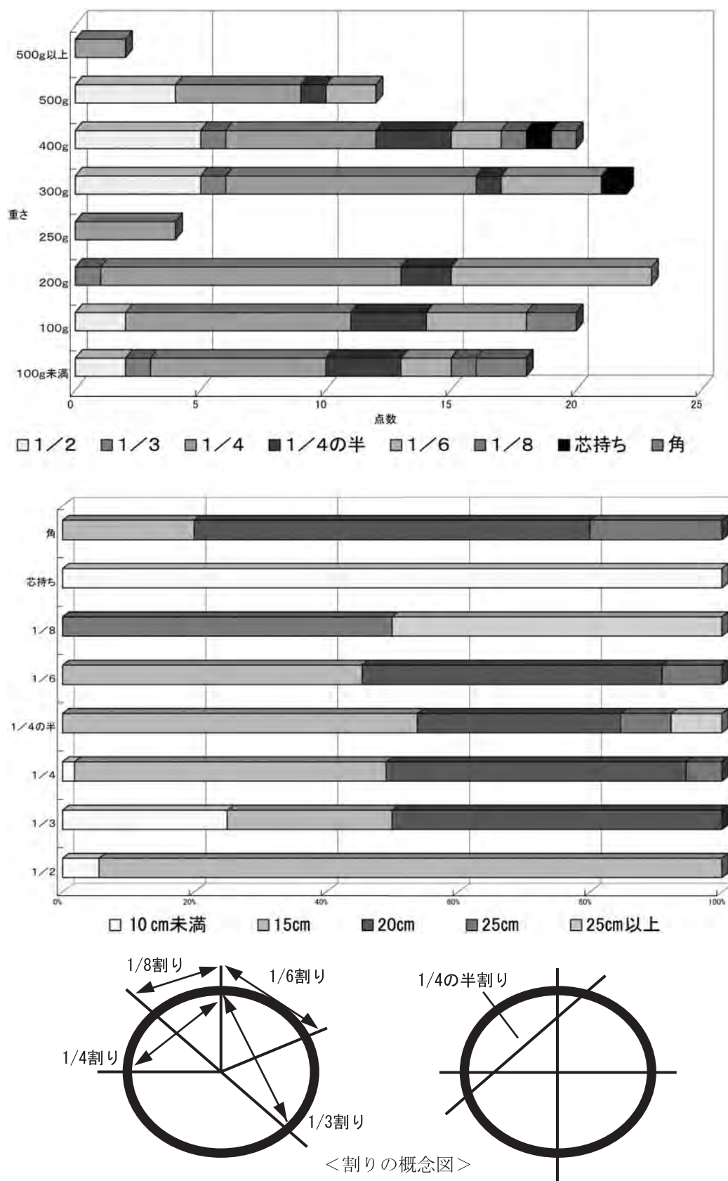
図10 木炭の小割りと重さ及び推定直径
