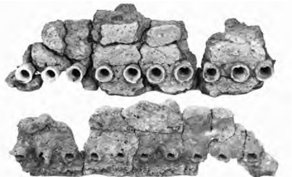
写真12 山田A遺跡出土炉壁装着羽口
