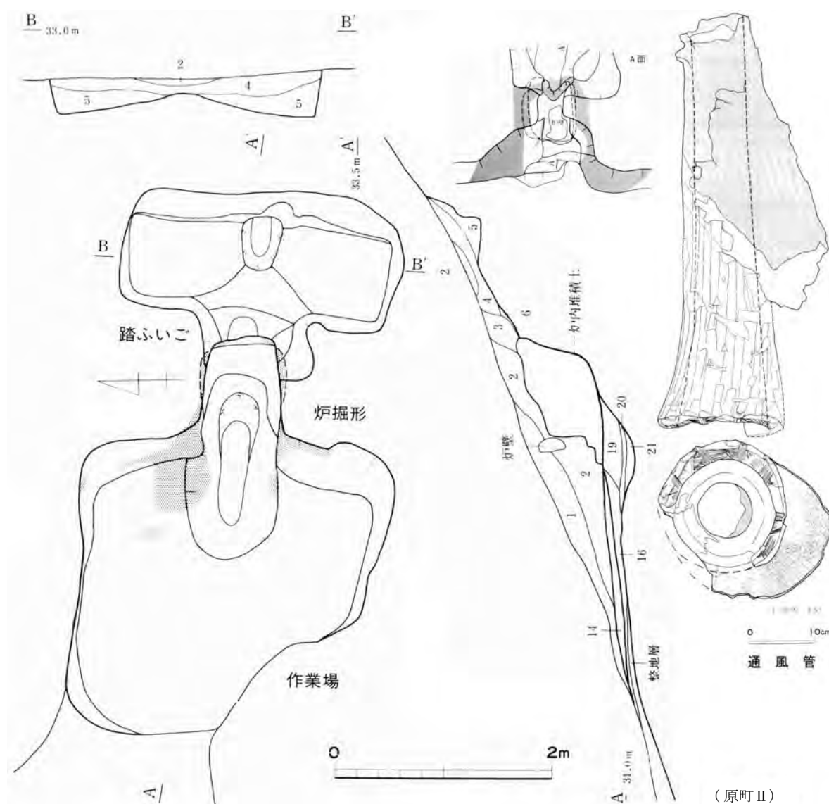
図 10 長瀬 3 号製鉄炉跡
