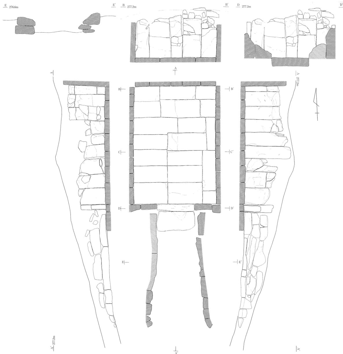
図3 稲古館古墳 横穴式石室展開図
