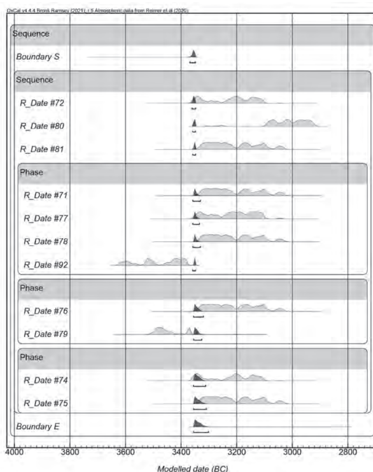
第3図 層序の ^{14}\text{C} ベイズ推定解析
