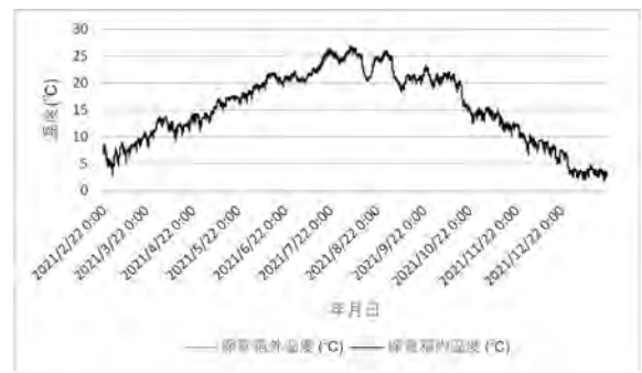
第7図 保管箱内温度と外部温度の変動比較
