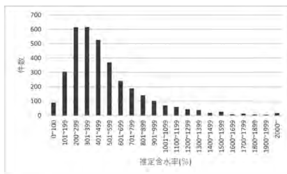
第12図 保管木質遺物含水率
