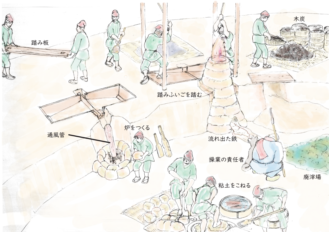
国指定史跡「横大道製鉄遺跡」8世紀中葉頃の竪形炉操業推定図
